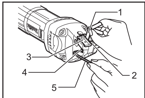
► 1. Gabarit d'épaisseur 2. Lame centrale 3. Lame latérale 4. Boulon à tête creuse hexagonale 5. Clé hexagonale
