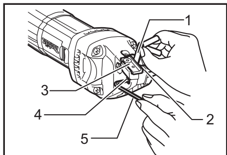
► 1. Calibrador de grosor 2. Superficie de cuchilla central 3. Cuchilla lateral 4. Perno hexagonal de la cabeza de conexión 5. Llave hexagonal
